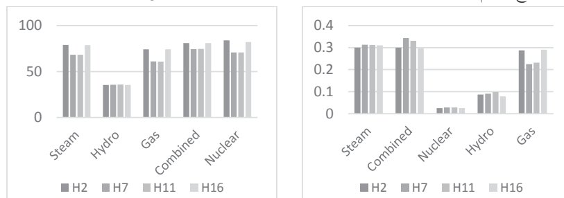
نمودار ۶- آثار اجرای سناریوی MCP بر متغیرهای هدف
