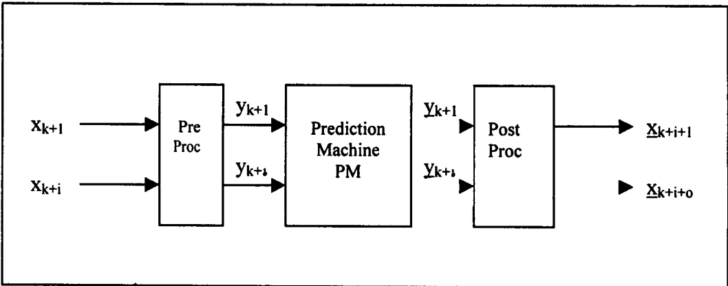
شکل - ۶. روش سوم پیش‌بینی
